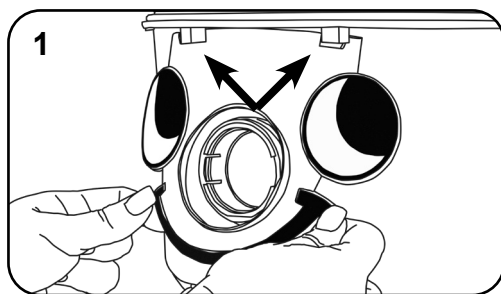
Removing the Face - Entfernen des Gesichts - Démontage du visage - Het gezicht verwijderen - Retirar a cara - Smontaggio frontale - Desmontaje de la cara - Zdejmovanie obudowy - Ta bort ansiktet - Etupaneelin irrottaminen - Afmontering af hovedet
